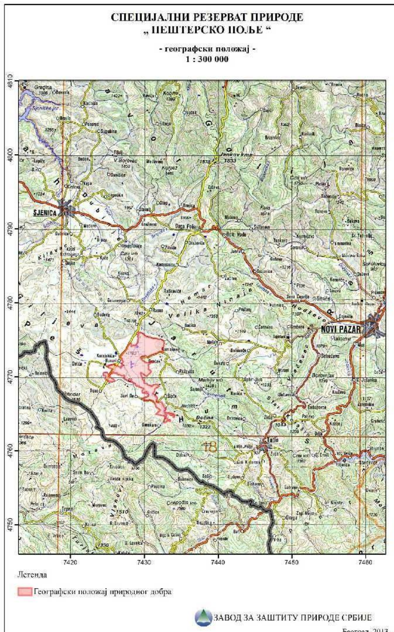
Географски положај СРП „Пештерско поље“
