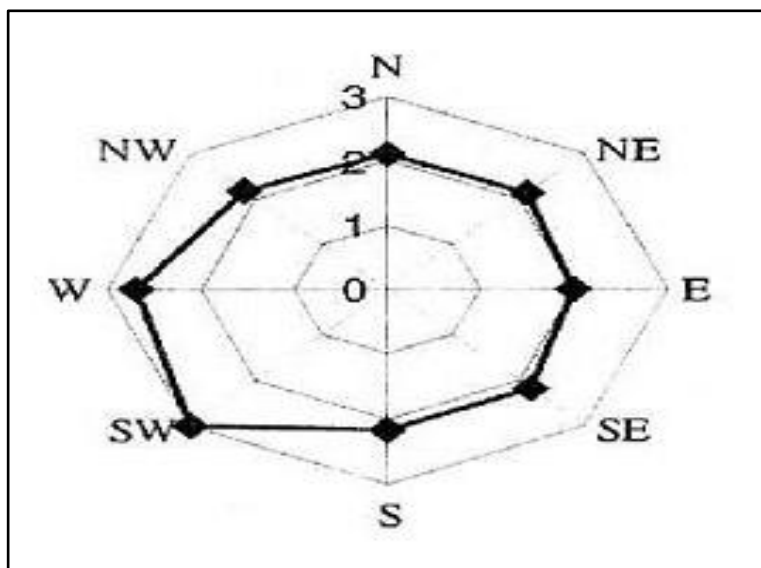
Јачине ветрова у Сјеници
