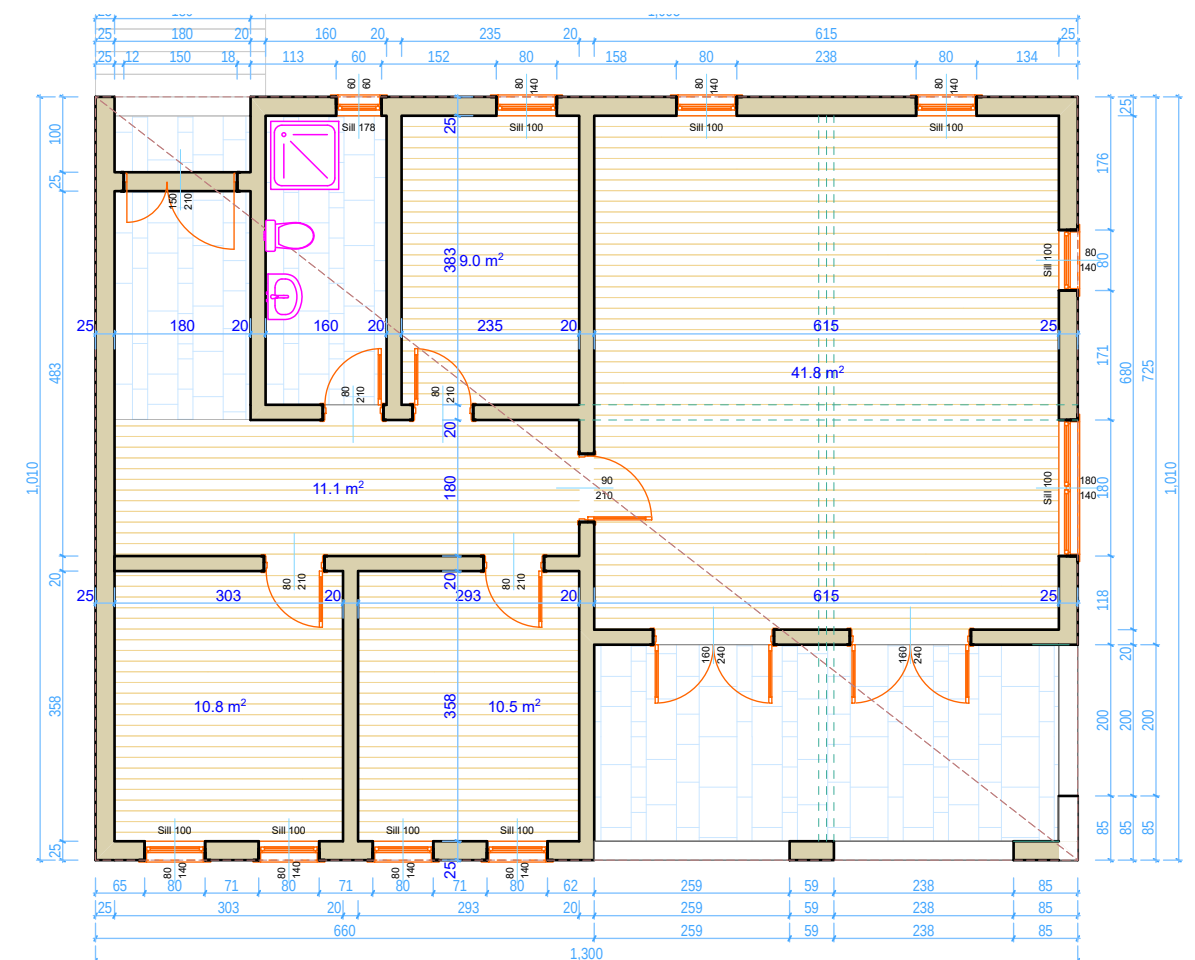
1. OSNOVA PRIZEMLJA 1:100
