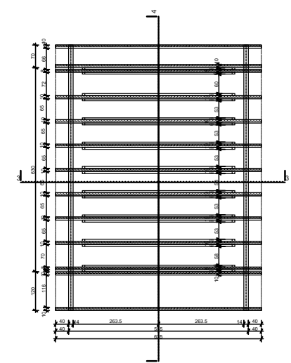
OSNOVA KROVNE KONSTRUKCIJE
