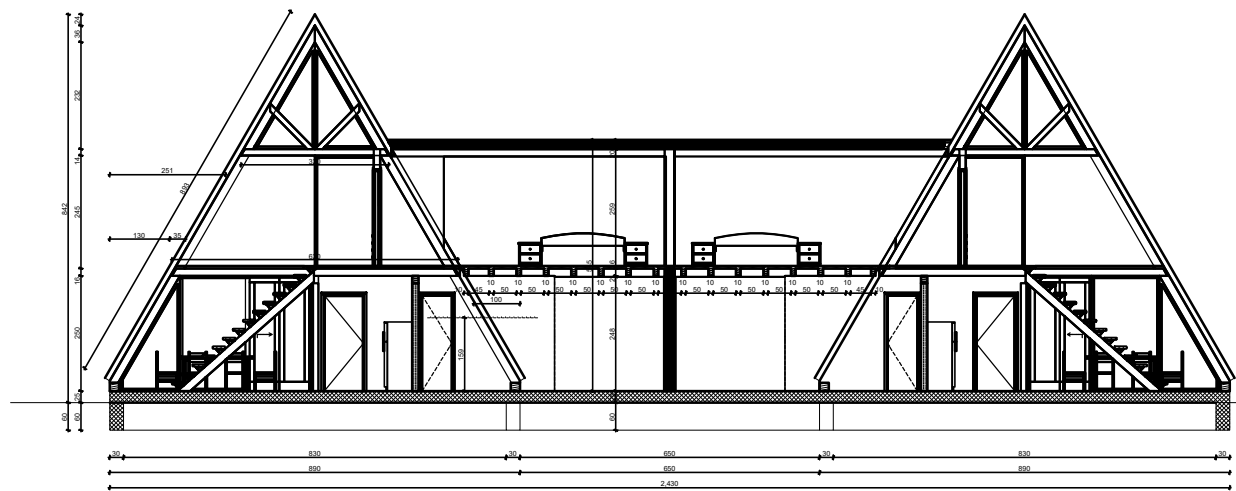
PRESJEK 1/1
