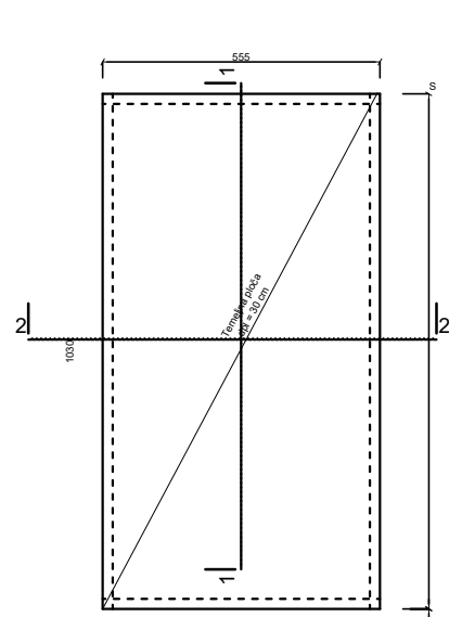
OSNOVA TEMELJA
