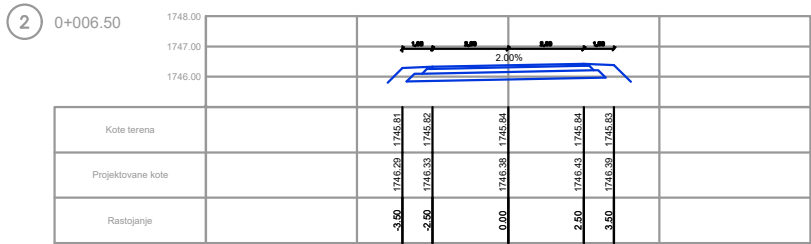
Poprečni profili priključka
