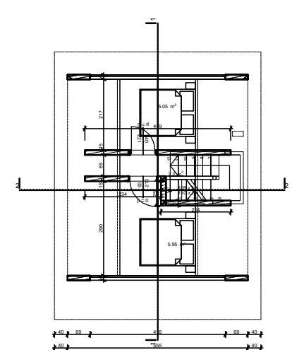
OSNOVA POTKROVLJA
