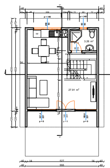
OSNOVA PRIZEMLJA
