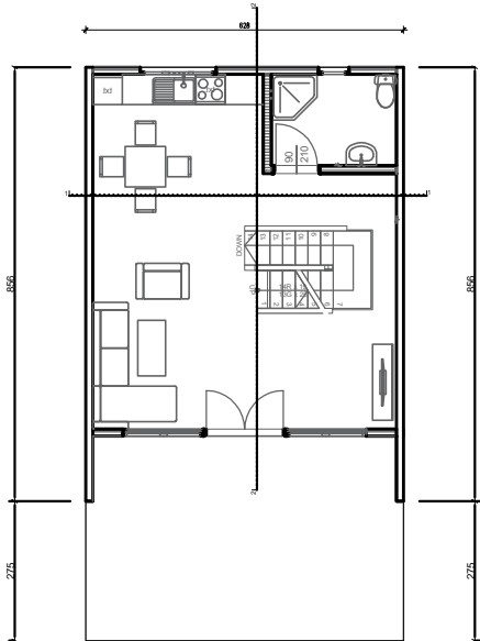
OSNOVA PRIZEMLJA
