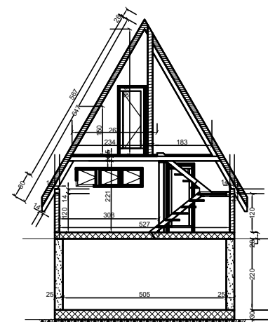
PRESJEK 2/2
