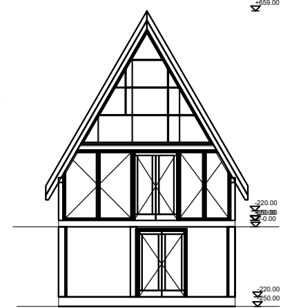
JUG-ZAP FASADA
