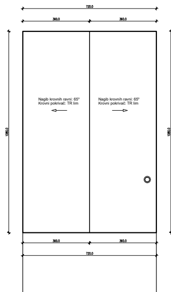
PETA FASADA
