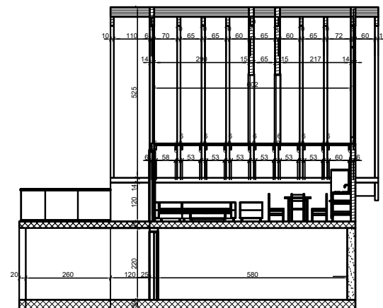
PRESJEK 1/1
