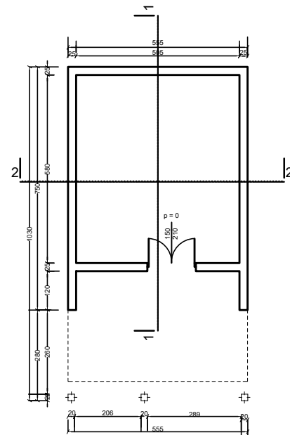
OSNOVA SUTERENA
