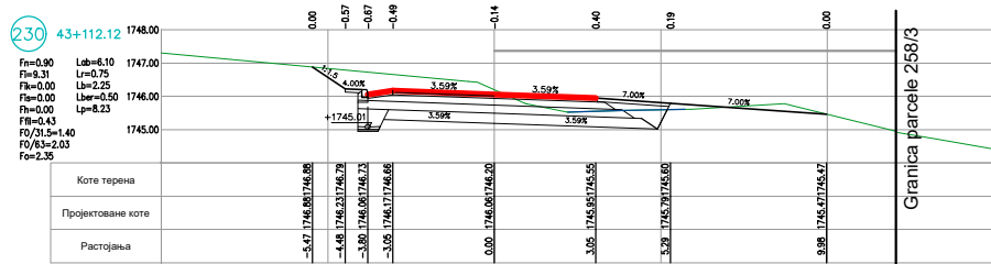
Poprečni profili državnog puta IIA br.198
